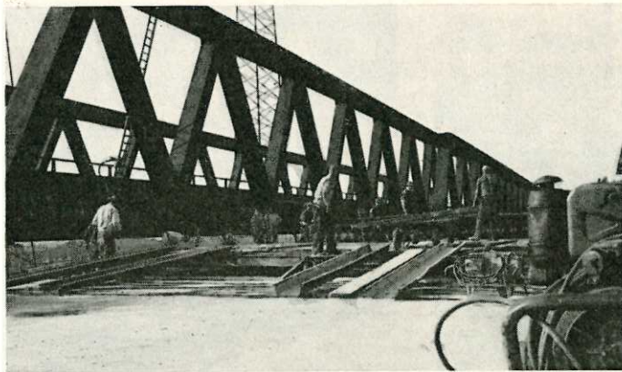
Das linke Bild zeigt die Brücke im Zuge der B 51 über Rhein-Herne-Kanal, Emscher und Zechenplatz der Zeche Recklinghausen I/II, wo auch noch die Bundesbahnstrecke Wanne—Recklinghausen überquert wird. Zu sehen ist die Stahlkonstruktion für die Brücke, die noch auf ihre richtige Höhe abgesenkt werden muß.
