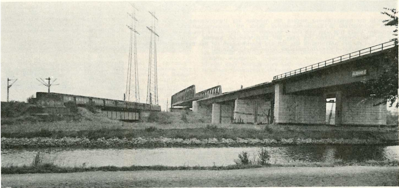
Das rechte Bild zeigt die beiden voneinander getrennten Fahrbahnen dieses Brückenzuges in seinem Abschnitt über den Rhein-Herne-Kanal mit Blickrichtung nach Baukau und zur Stadt zurück. — Das letzte Bild unserer Wanderung über die Trasse der künftigen Bundesstraße 51 neu von der Stadtgrenze Herne—Bochum bis zum Rhein-Herne-Kanal zeigt den in den beiden vorigen Bildern von oben dargestellten Brückenzug aus der Sicht des am Rhein-Herne-Kanal stehenden Fußgängers. — Hier empfindet man, daß das, was noch vor zwei oder gar drei Jahren verkehrstechnische ferne Herner Zukunft war, dank eines verwirrenden und großartigen Zusammenspiels vieler Kräfte überraschend schnell Gegenwart geworden ist.
