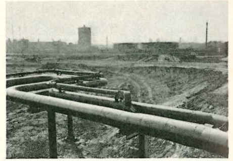
Blick auf die beginnende Dammschüttung für den Auffahrtsarm B 51/Eickeler Straße. Im Vordergrund Rohrleitungen der Hibernia, die durch das Bauwerk im Zuge der Eickeler Straße über die Zechenbahn bereits verlegt wurden. Im Hintergrund die Anlagen der Hibernia-Chemie.
