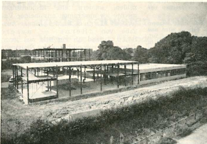
Das Stahlskelett der Schule nach der Vollendung der Montagearbeit. Nur diese Bauweise konnte der Zeitnot gerecht werden. (Werkfoto: Krupp)
