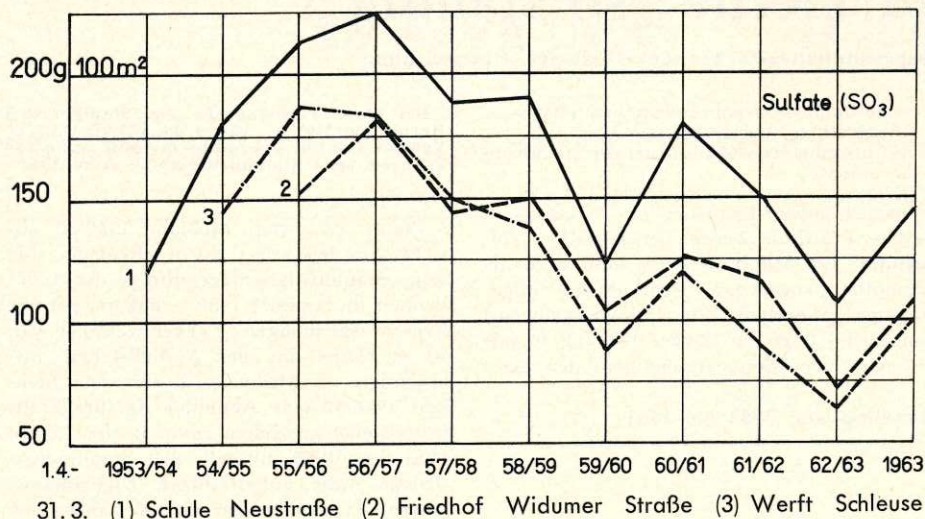
mittlerer monatlicher Sulfatniederschlag von 1953 bis 1963
